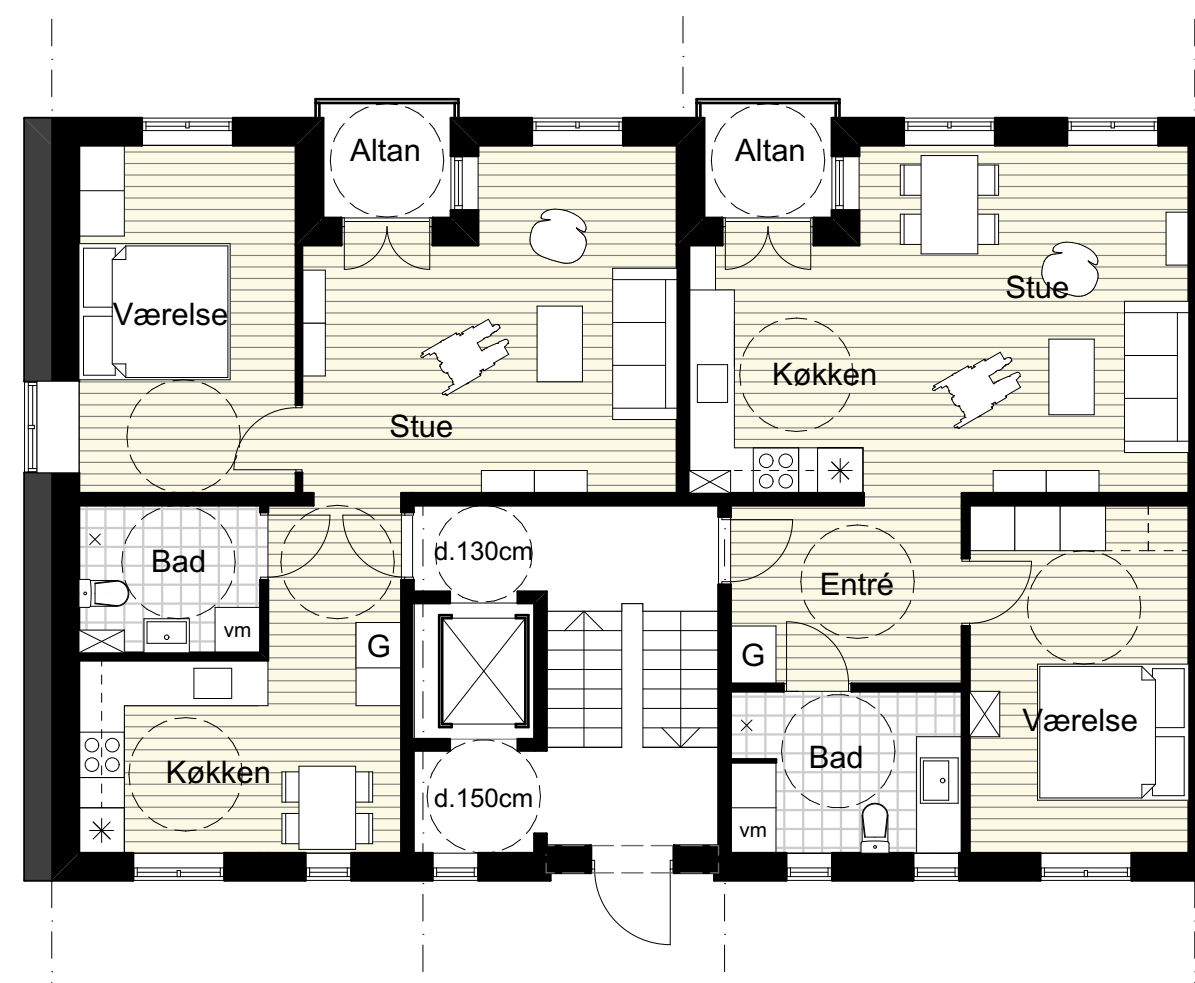
2v - tilgængelig bolig
